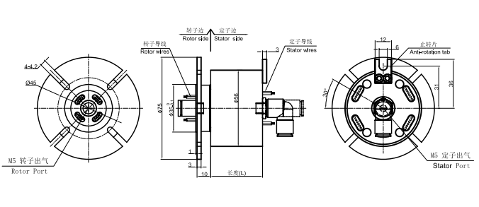
MAPH100-02 尺寸图
