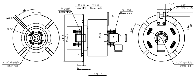
MAPH100-05 尺寸图
