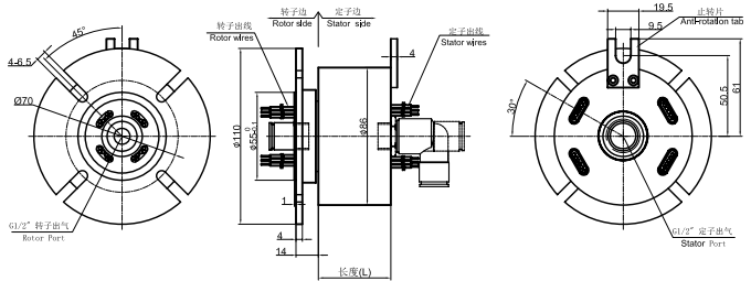
MAPH100-05 尺寸图
