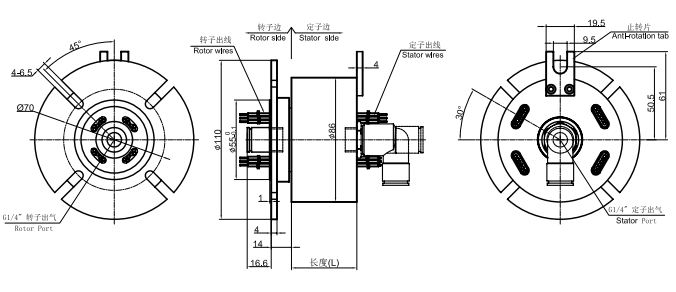
MAPH100-03 尺寸图
