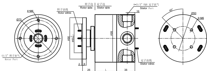
MAPH104-05 尺寸图
