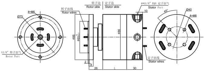
MAPH104-02 尺寸图
