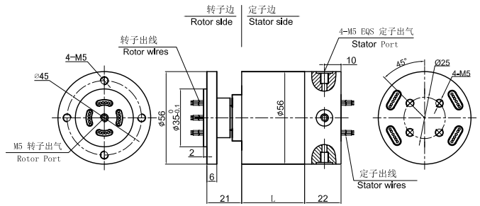
MAPH104-02 尺寸图
