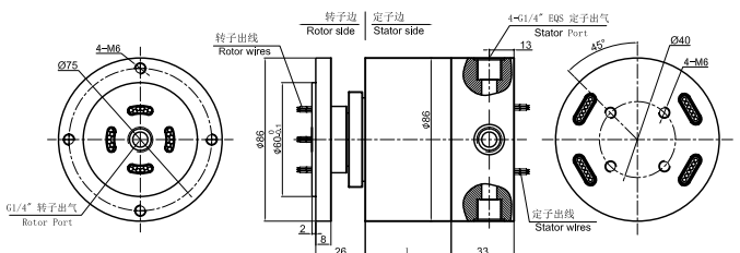
MAPH104-03 尺寸图
