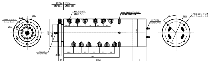
MAPH1200-01 尺寸图
