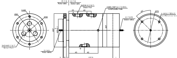
MAPH300S-03 尺寸图
