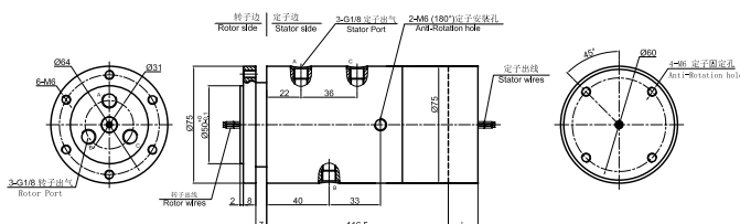
MAPH300S-03 尺寸图
