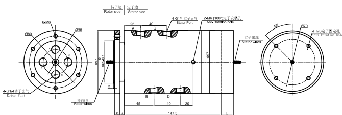
MAPH400S-03 尺寸图
