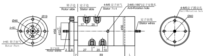
MAPH400S-01 尺寸图
