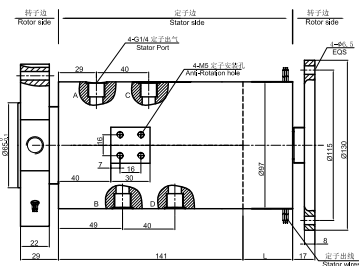
MAPH400W-03 尺寸图
