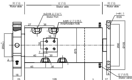
MAPH400W-03 尺寸图
