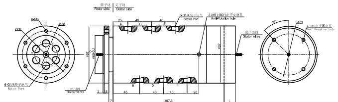
MAPH600S-03 尺寸图
