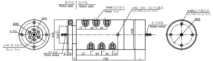
MAPH600S-02 尺寸图
