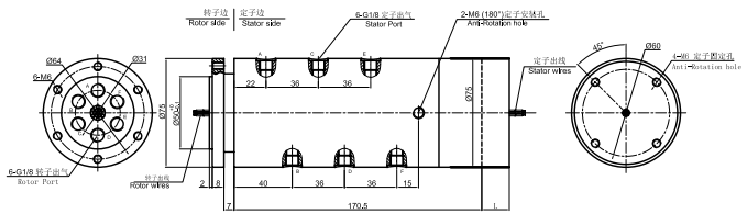
MAPH600S-03 尺寸图
