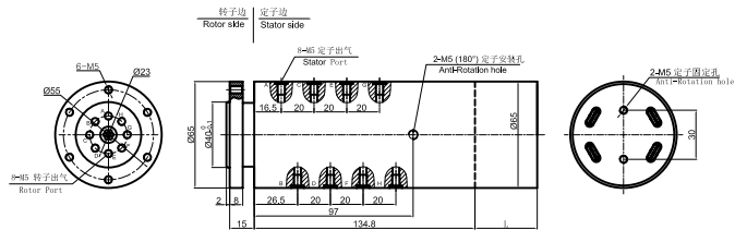
MAPH800-02 尺寸图
