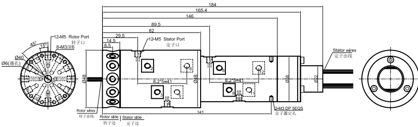
MQR12-S24 尺寸图 12进12出, M5牙 + 24路信号(2A)
