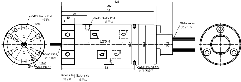
MQR6-S24 尺寸图 6进6出, M5牙 + 24路信号(2A)
