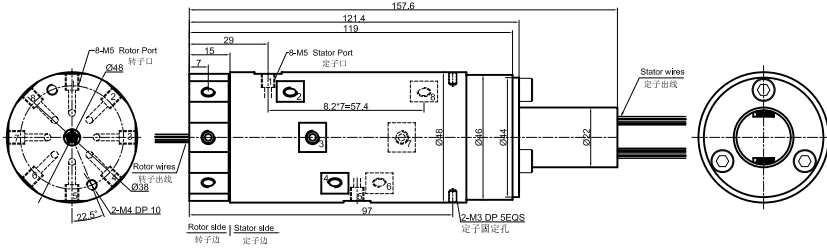
MQR12 尺寸图 12进12出, M5牙
