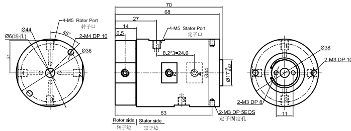
MQR4-S12 尺寸图 4进4出, M5牙 + 12路信号(2A)
