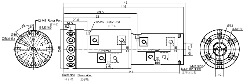
MQR12-S12 尺寸图 12进12出, M5牙 + 12路信号(2A)
