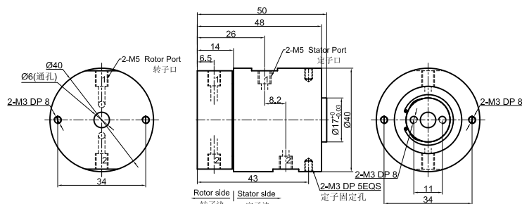
MQR2 尺寸图 2进2出, M5牙
