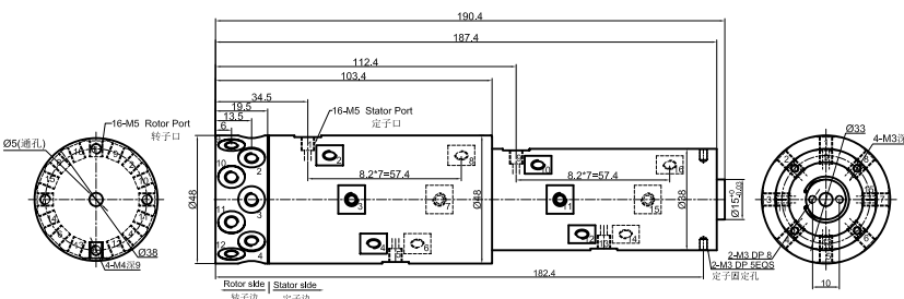
MQR16 尺寸图 16进16出, M5牙
