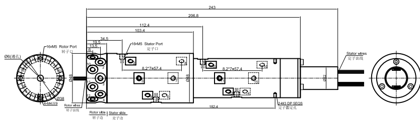
MQR16-S24 尺寸图 16进16出, M5牙 + 24路信号(2A)
